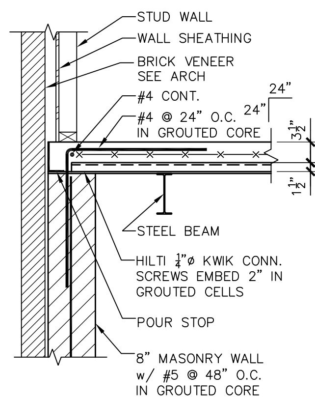
SECTION 4 SCALE: 3/4"=1'-0"
