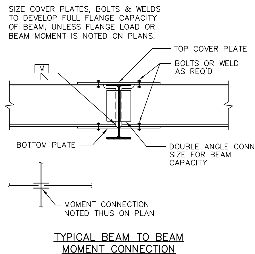
SECTION 8 SCALE: 3/4"=1'-0"
