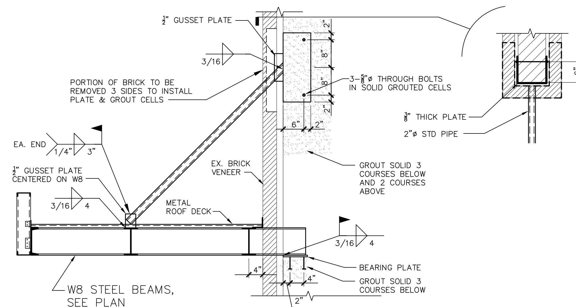
SECTION 10 SCALE: 3/4"=1'-0"
