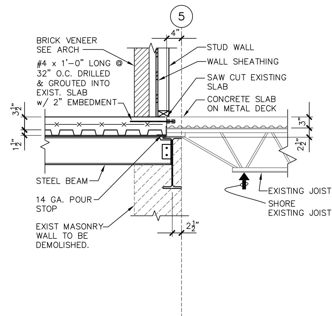
SECTION 5 SCALE: 3/4"=1'-0"
