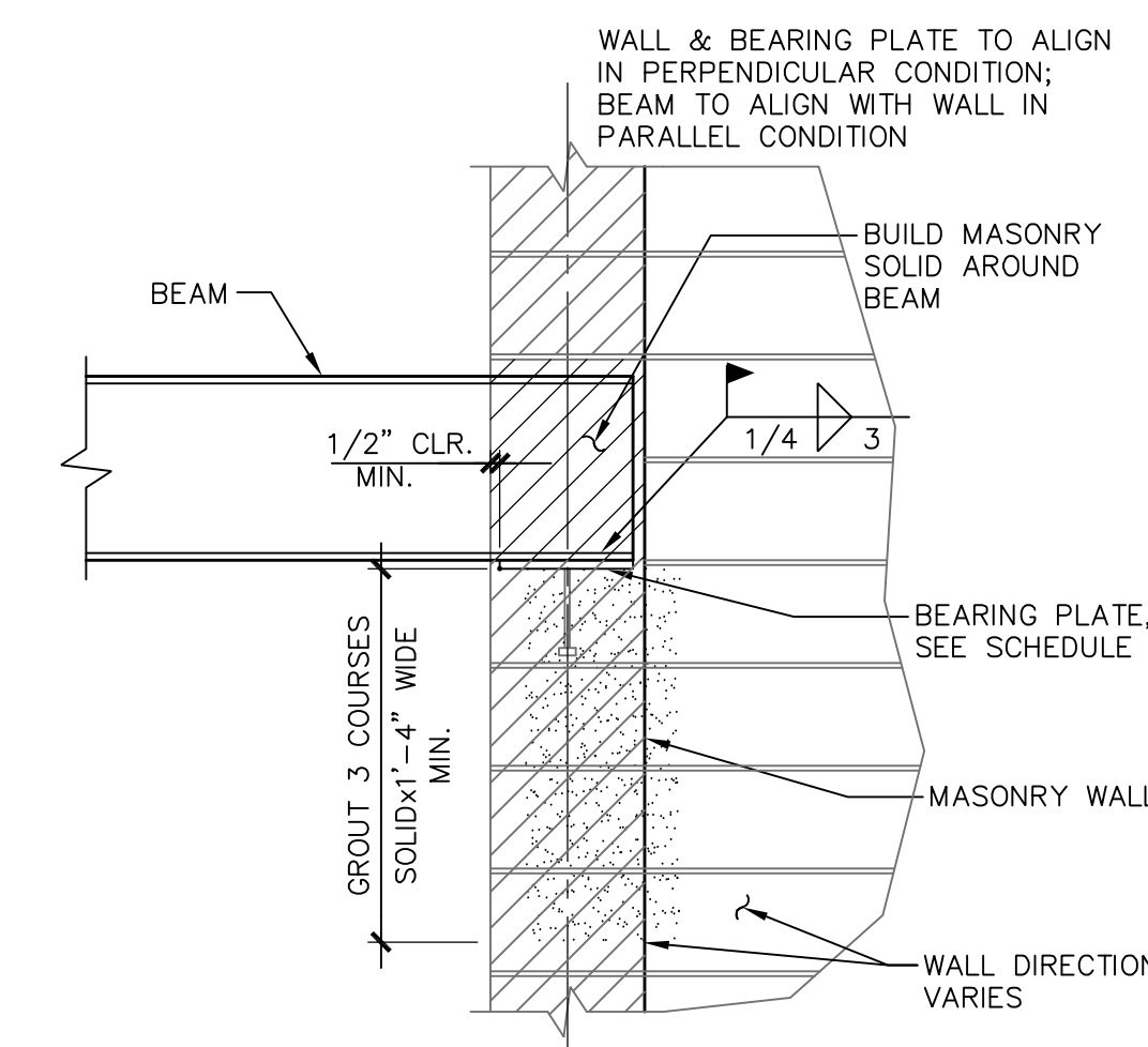
SECTION 6 SCALE: 3/4"=1'-0"
